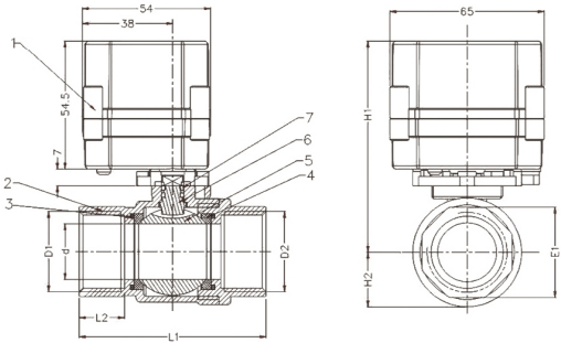
Assembly Diagram 组装图
